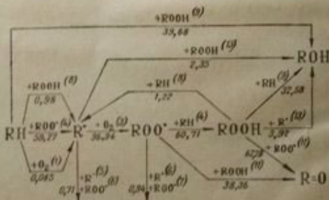
Рис. 3. Расчетный механизм жидкофазного окисления толуола (Цифры под стрелкой указывают долю распадающего вещества в данном направлении в %).
