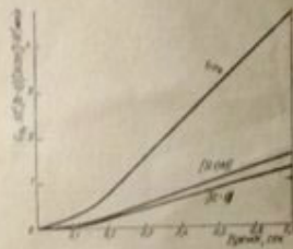
Рис. 2. Расчетные кинетические кривые накопления R-O и ROH в присутствии O₂.
