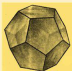
Додекаэдр
