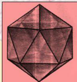
Икосаэдр
