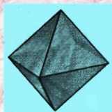
Октаэдр
