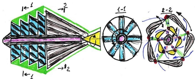
Рис. 13. Вихревой движитель
