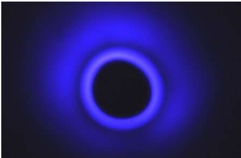
Рис. 32. Вихрь «икринки» плазмы как «точка роста» (Habr)
