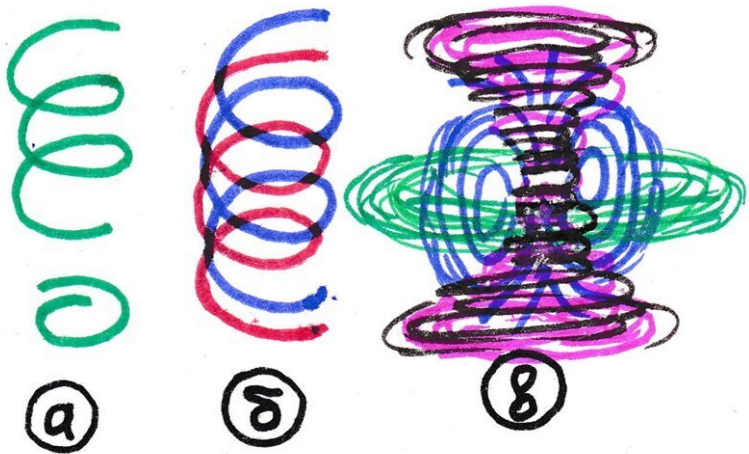
Рис. 2. «а» – «одионый нулевой» вихрь, «б» – двойная спираль вихрей «а» одного спина, «в» – «нулевой» диполь
