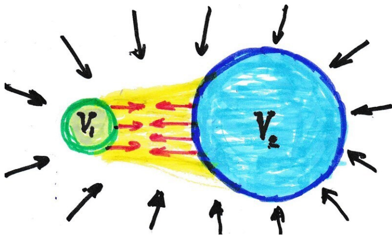
Рис 4. Теория теней двух объектов гравитации ЛеСажя
