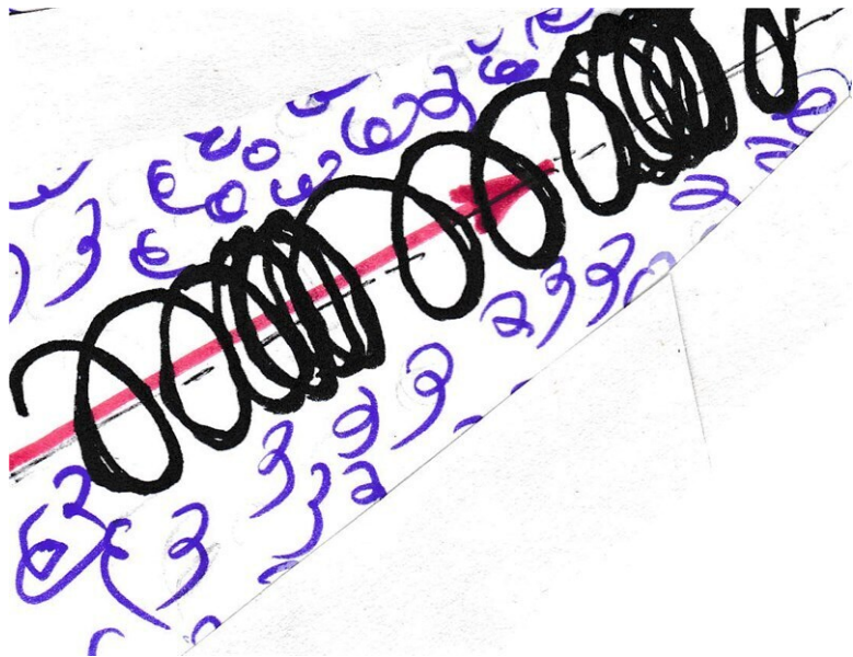
Рис. 28. Звук как результат взаимодействия вихрей материи среды
