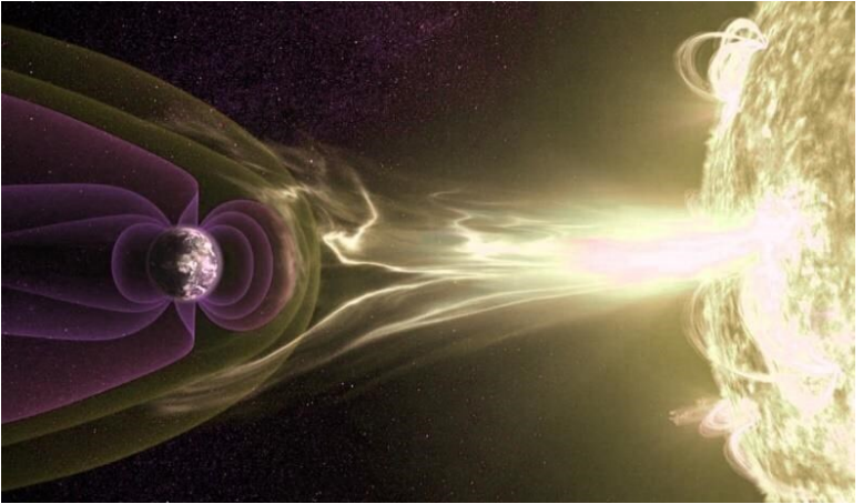
Рис. 5. Поток солнечной плазмы (фотошоп)
